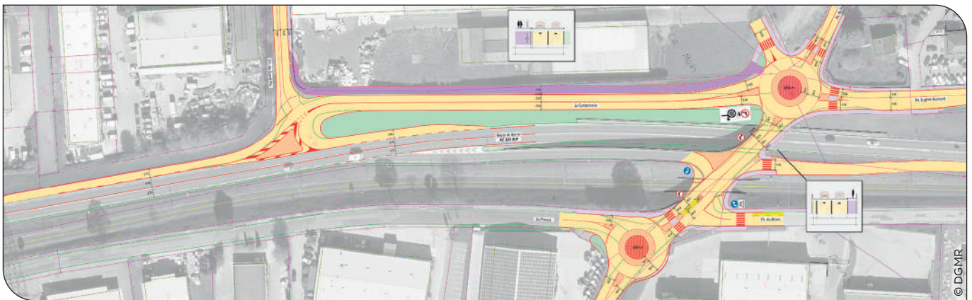
Plan de situation de la jonction sud avec la route de Berne
