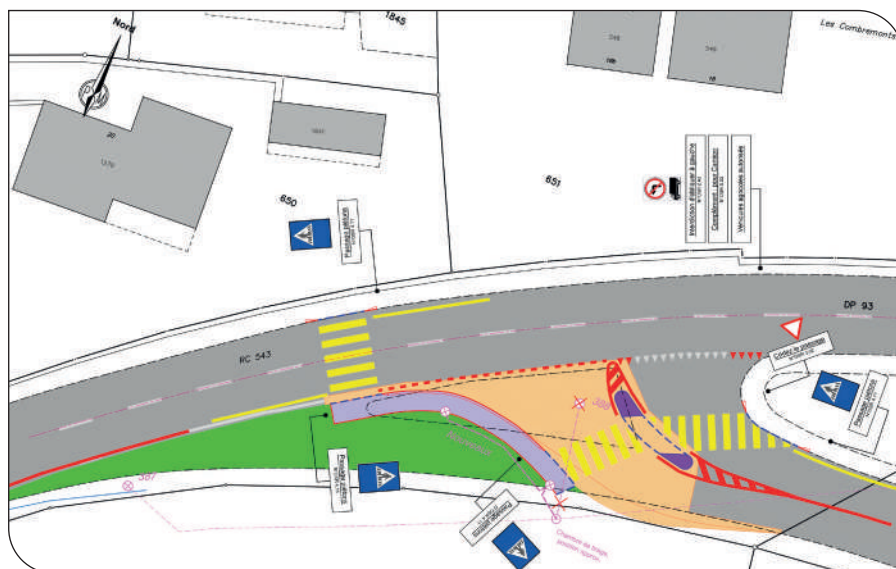
Plan du futur carrefour
